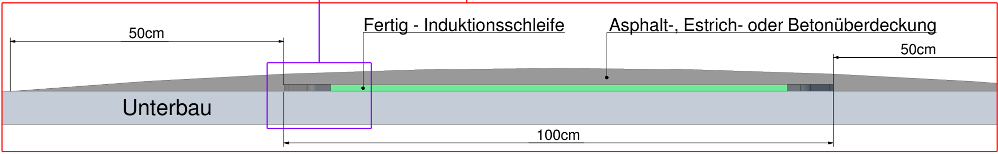
Befestigung der Fertig-Induktionsschleife auf dem Untergrund
